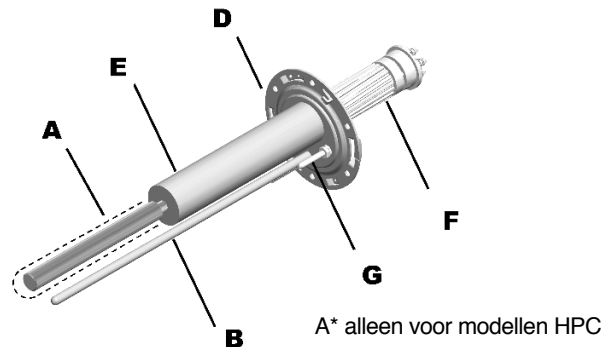
Afbeelding 3 – Weerstand steatiet + PROfessional TECH anode
